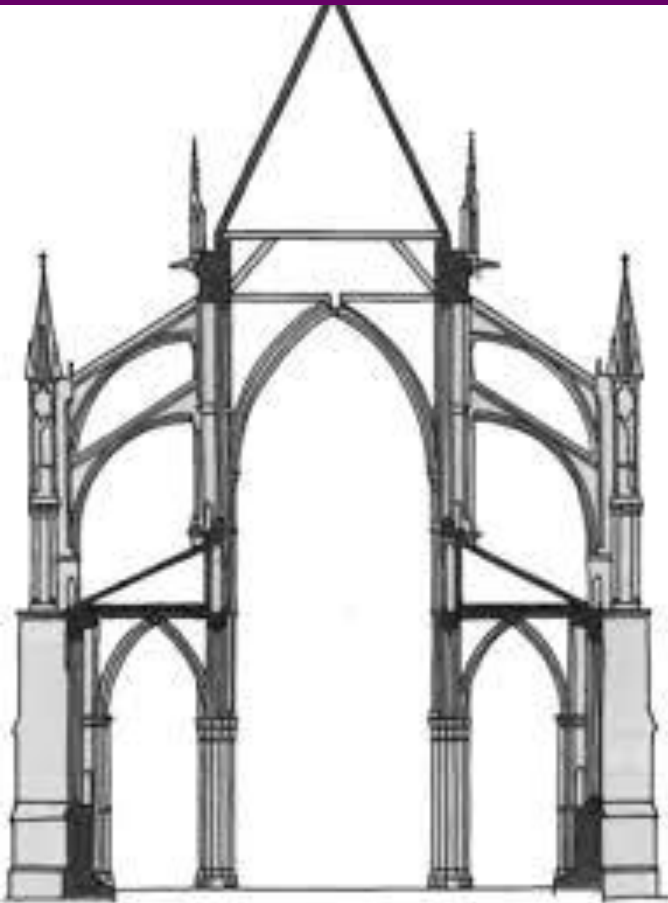
Поперечний розріз готичного храму.
